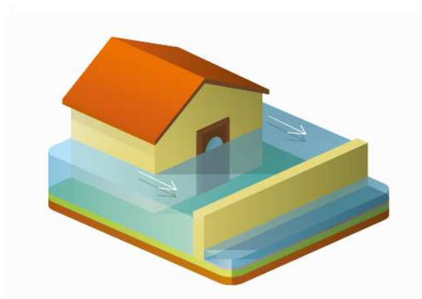
Figure 4: Exemple de clôture qui n'assure pas la transparence hydraulique. Source : Mayane pour la DDT du Bas-Rhin, 2017
