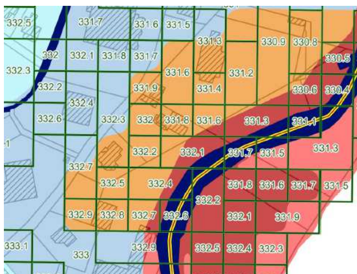
Figure n°6 : Extrait de la planche 03 (les CPHE* représentées n'incluent pas la revanche de 0,30 mètre)
