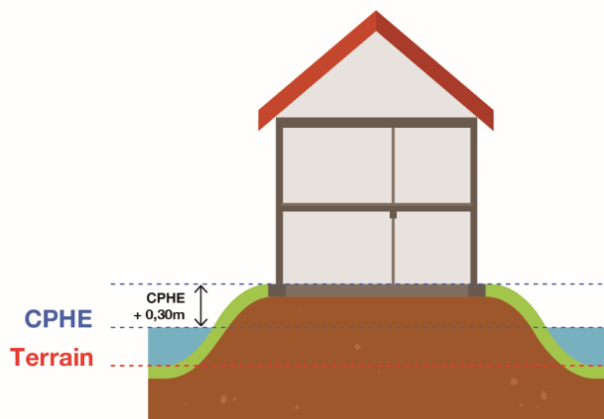
Figure n°7: Illustration de l'implantation d'un bâtiment en zone de débordement de cours d'eau
