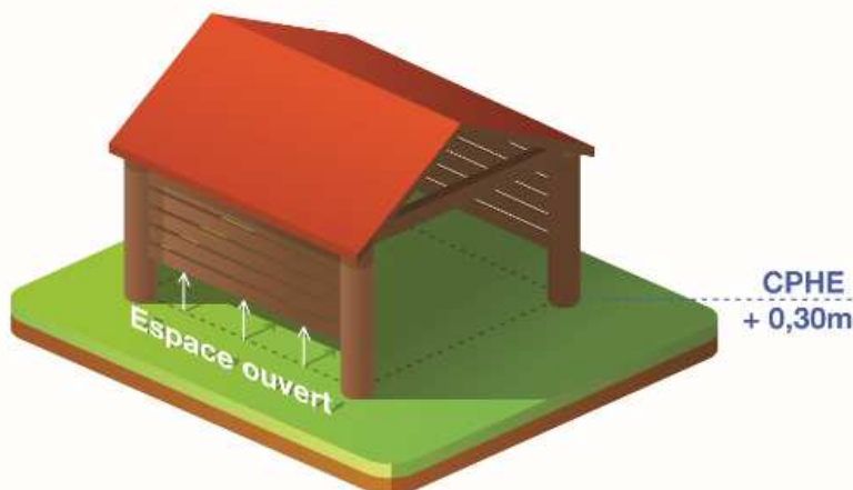
Figure 5: Illustration d'un bâtiment ne comportant pas de paroi sous la CPHE
